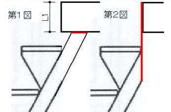
梁の場合の取付方法 赤線は上部プレートを視す
